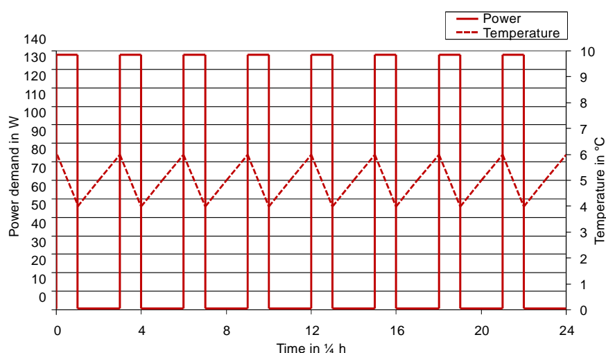
Abbildung 3-1: Generelles Verbrauchsmuster eines Kühlschranks
