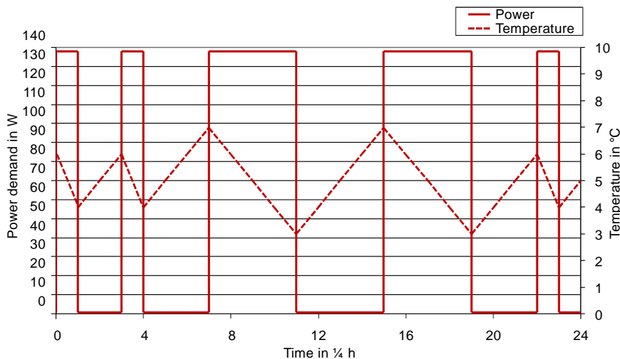
Abbildung 3-2: Generelles Verbrauchsmuster eines Kühlschranks mit verlager-tem Start des Kompressors
